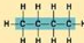
Butane
