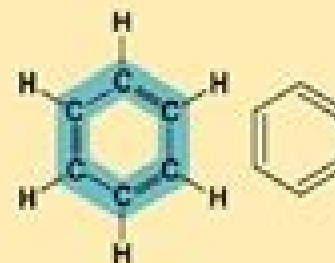
Benzene
