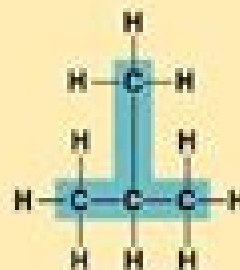
Isobutane
