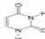
Uracil
