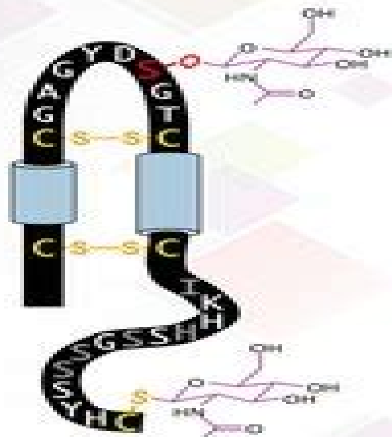
Glycocin F
