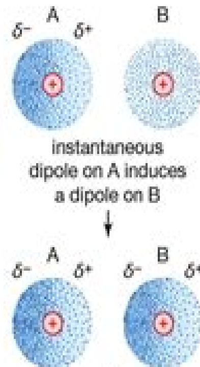
van der Waals bond
