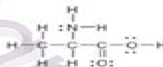
C_3H_7NO_2
