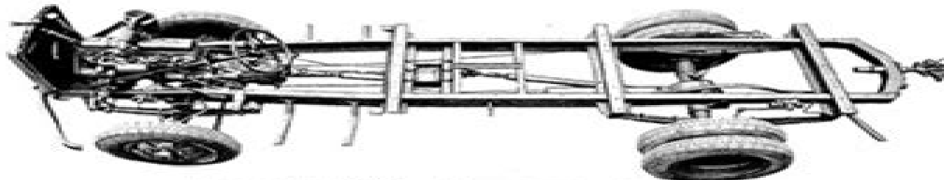
Fahrgestell 6700 Typ A nur in Wehrmachtausführung
