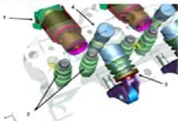
Fig. 5 Modulo MultAir (sezione per singolo cilindro)
